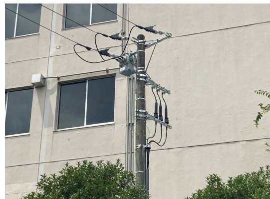
高圧気中開閉器(構内引込柱に設置)
